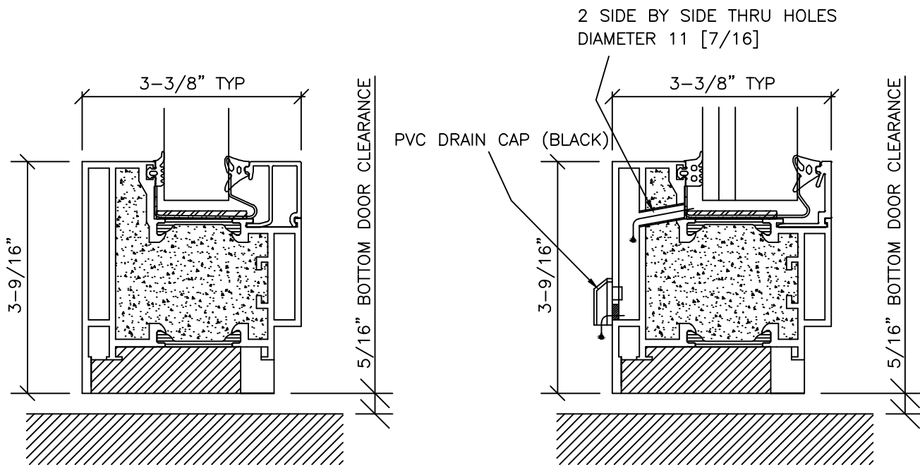
4 BOTTOM DOOR RAIL SECTION 60 MIN. GLASS
